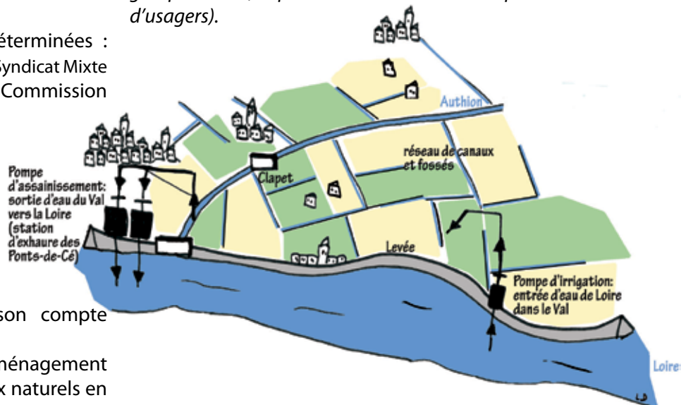
Représentation simplifiée des ouvrages hydrauliques sur le val d'Authion et du Lane
